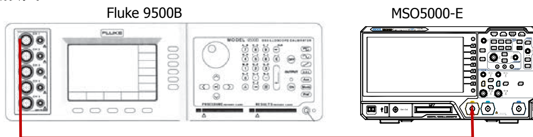
图 2-3 带宽测试连接图
