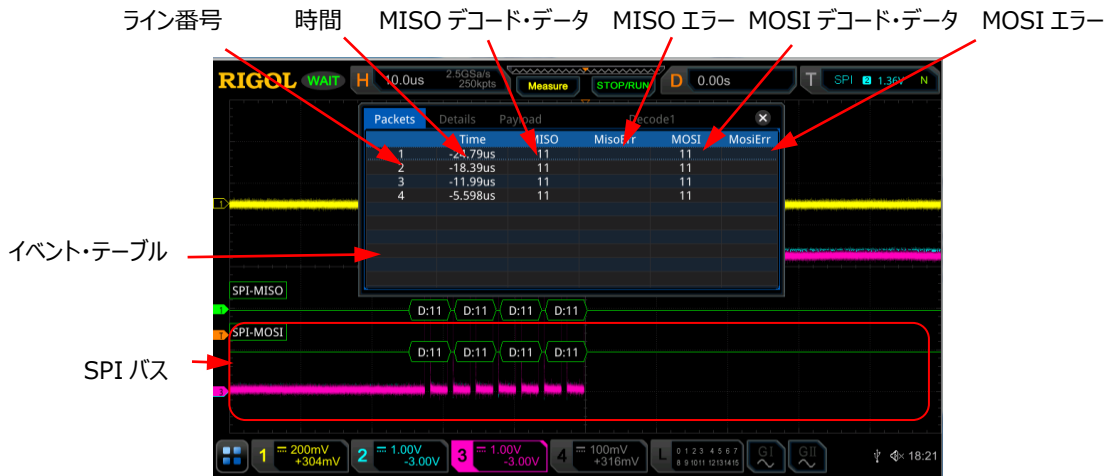
Figure 11-8 SPI デコード・イベント・テーブル
