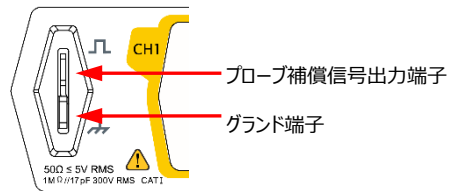
Figure 1-10 プローブ補償信号を使用する
