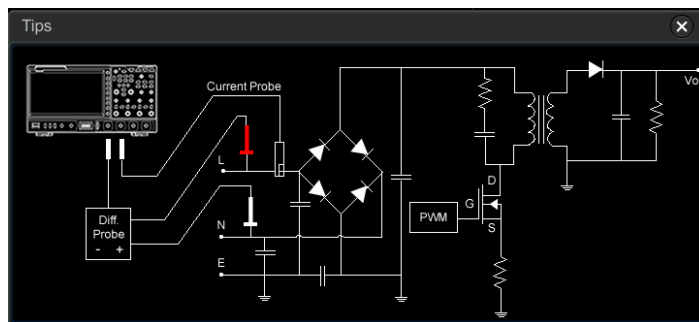
Figure 8-1 パワー・クオリティ解析の接続図
