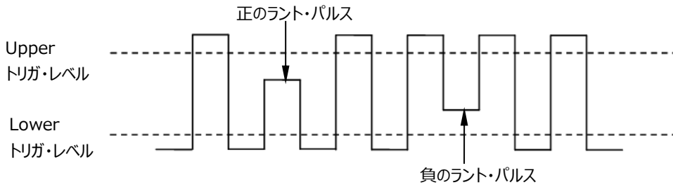
Figure 5-9 ラント・トリガ
