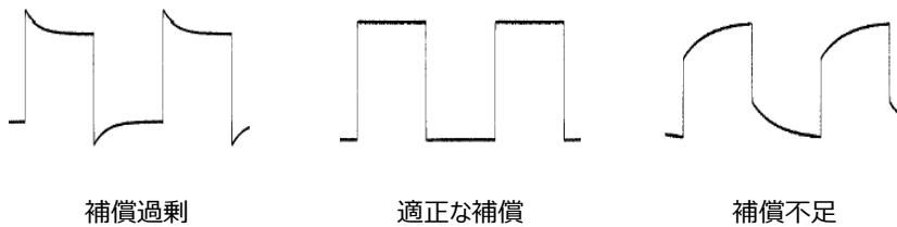
Figure 1-12 プローブ補償
