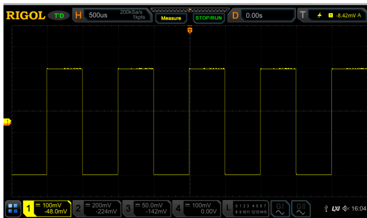
Figure 4-3 128 回アベレージした波形
