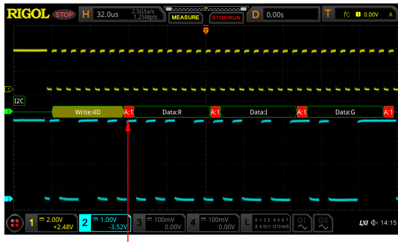
ACK が 1 であることを検出
