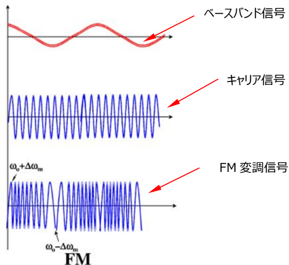
Figure 17-11 FM（周波数変調）
