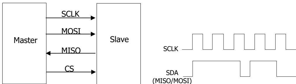
Figure 11-7 SPI シリアル・バス
