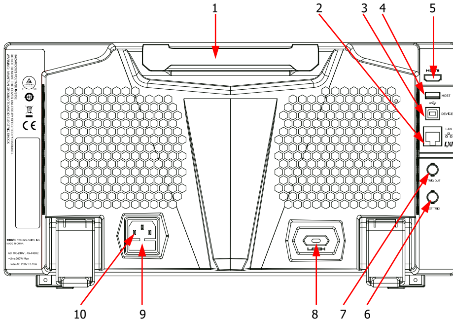
Figure 1-14 リア・パネル
