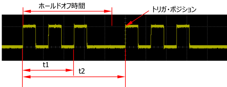
Figure 5-2 トリガ・ホールドオフ
