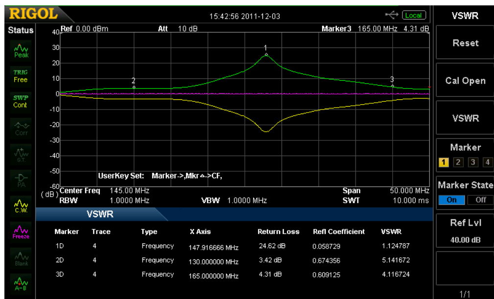
図 2-13 VSWR 測定画面
