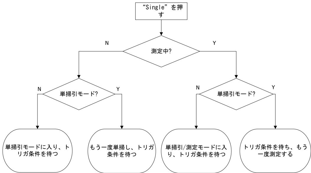
図 2-10 単掃引処理
