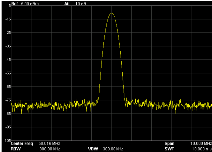
図 2-28 自動検出後
