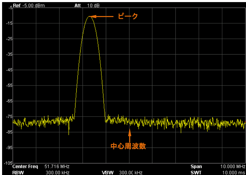
図 2-2 Peak->CF 実行前
