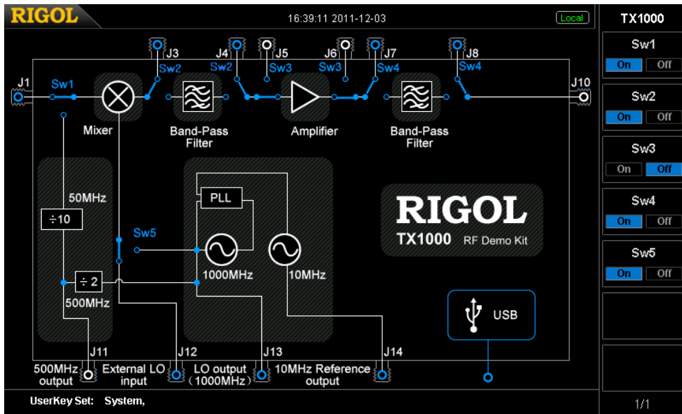
図 2-30 TX1000 コントロール パネル
