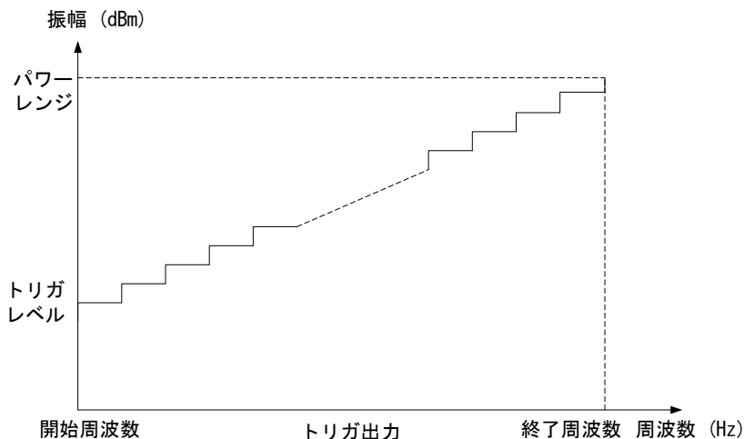
図 2-12 パワー掃引
